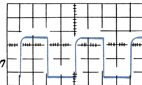
KT21 2 В/дел 10 мсек/дел
