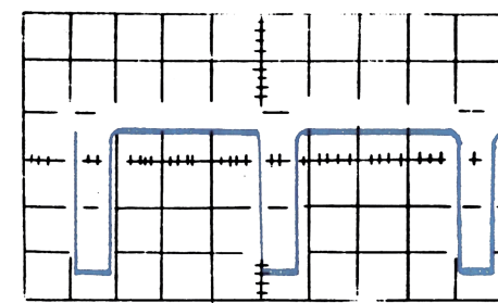
KT14 0,5 В/дел 5 мсек/дел
