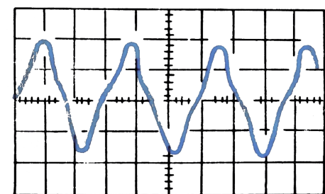
KT6 1 В/дел 0,1 мкс/дел
