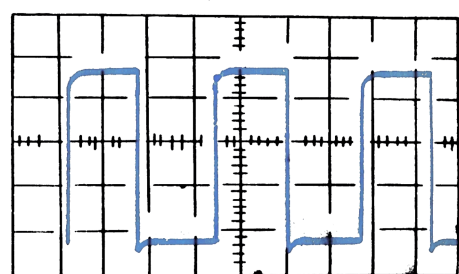
KT4 1 В/дел 5 мсек/дел
