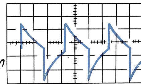
KT24 2 В/дел 20 мкс/дел
