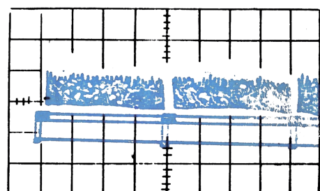
KT10 0,5 В/дел 5 мсек/дел
