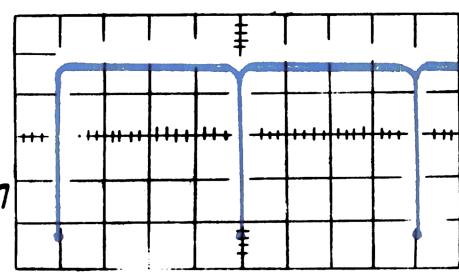
KT13 2 В/дел 10 мсек/дел
