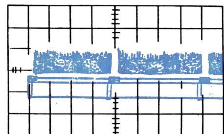
KT3 2 В/дел 5 мсек/дел
