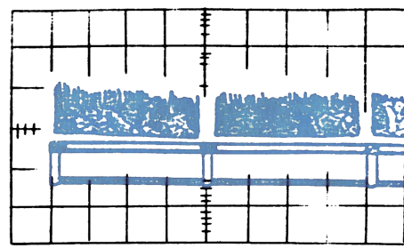
KT7 0,1 В/дел 5 мсек/дел
