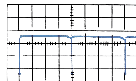
KT16 2 В/дел 5 мсек/дел
