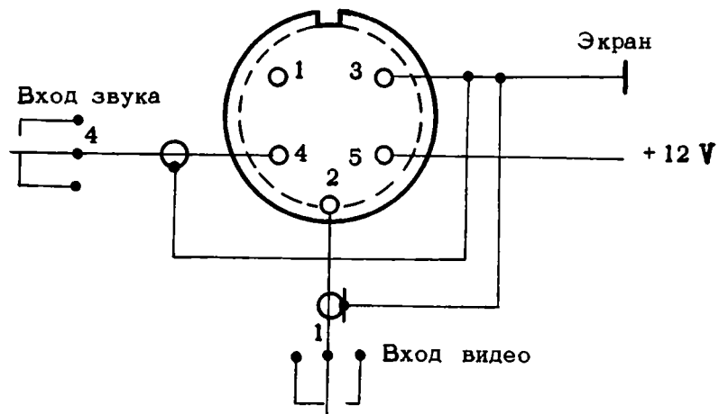
Рис.5. Сигналы на разъеме Ш5 в режиме "ЗАПИСЬ" "ТЕЛЕВИЗОР"
