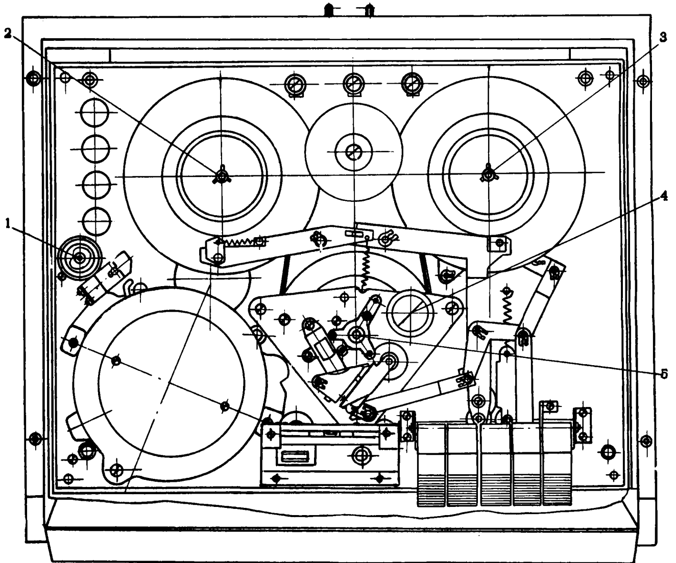
Рис. 64. Схема смазки:
