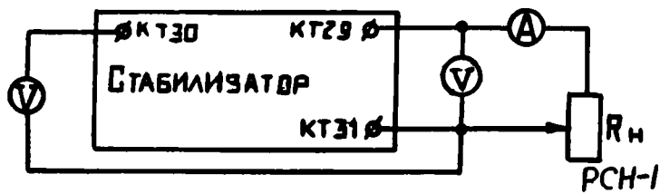
Рис. 32. Схема подключения
