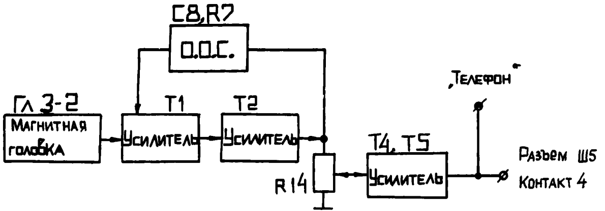
Рис. 18. Блок-схема канала звукового сопровождения в режиме "ВОСПРОИЗВЕДЕНИЕ"
