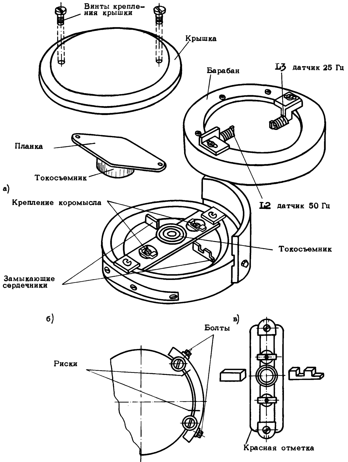
Рис. 30. Блок видеоголовок:
