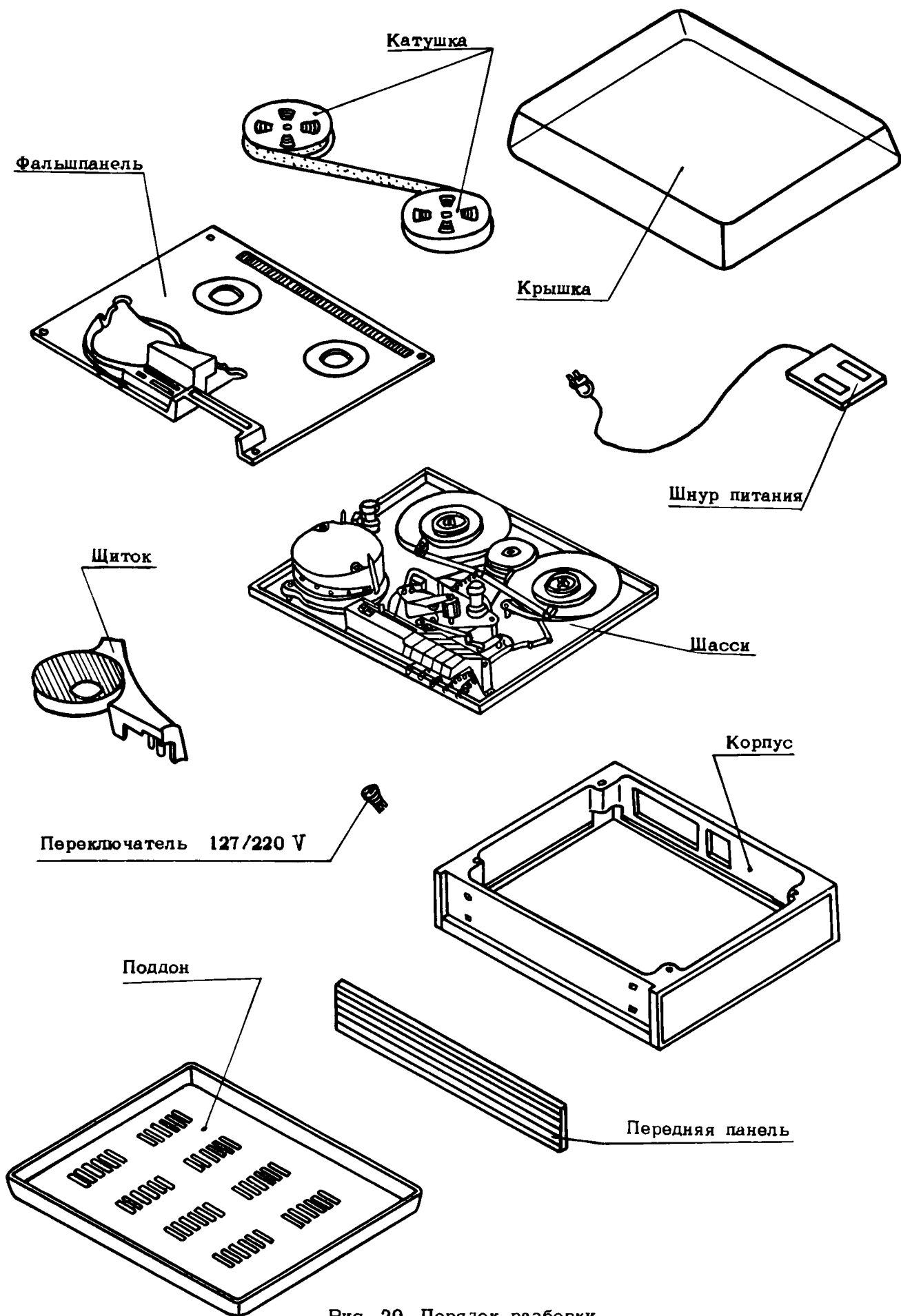
Рис. 20. Порядок разборки
