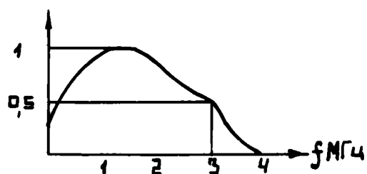
Рис. 59. Характеристика фильтра нижних частот платы 2
