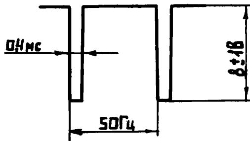
Рис. 49. Кадровые импульсы для синхронизации камеры в КТ23
