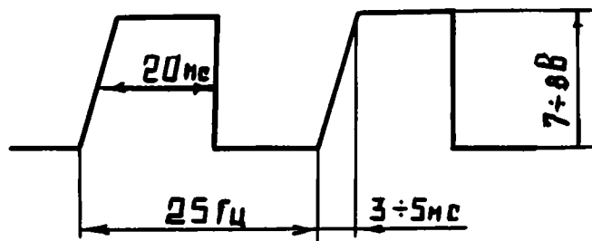
Рис. 34. Сигнал в КТ17
