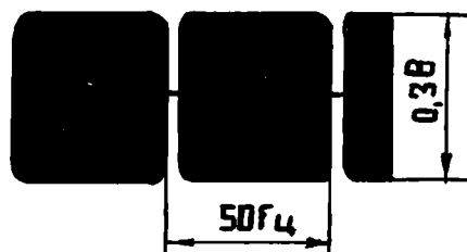
Рис. 43. Сигналы в КТ7 при неправильной установке датчика 50 Гц
