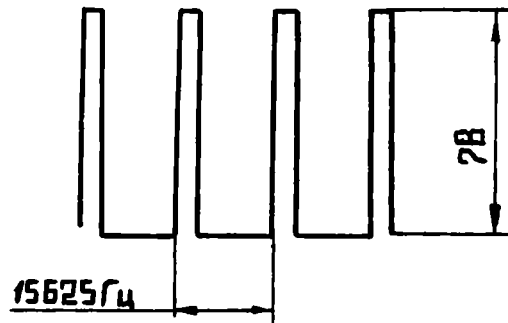
Рис. 37. Строчные синхроимпульсы в КТ15
