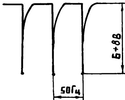
Рис. 38. Кадровые синхроимпульсы в КТ16
