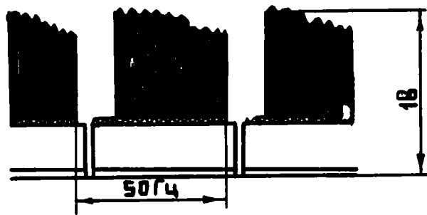
Рис. 33. Видеосигнал
