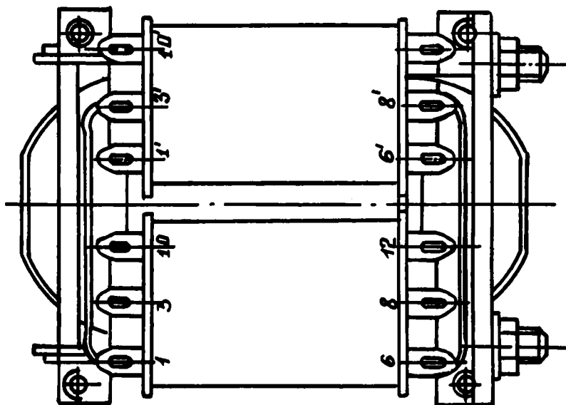
Рис. 71. Схема распылки трансформатора ТС-40
