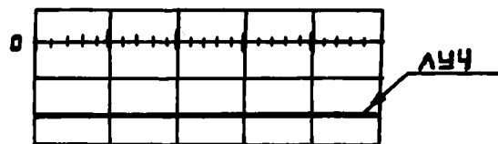
Рис. 53. Уровень напряжения на движке R30, соответствующий частоте модулятора 3,2 МГц
